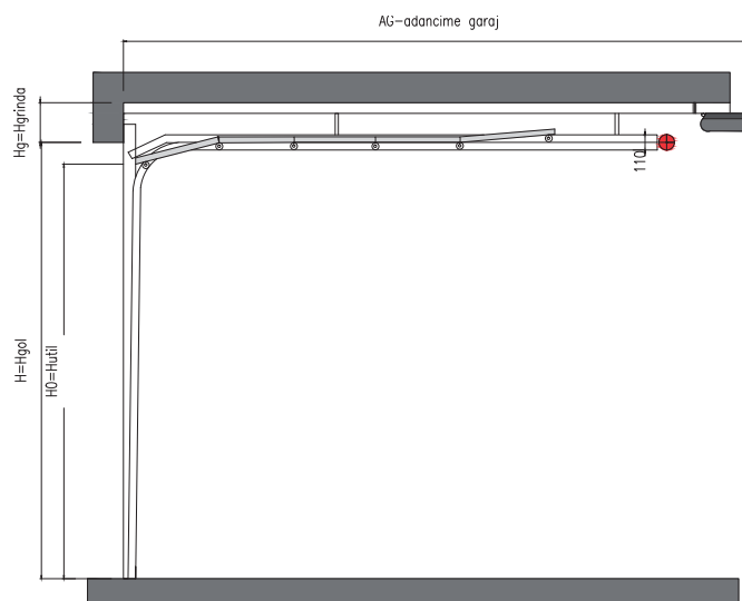
SECȚIUNE VERTICALĂ UȘA SECȚIONALĂ MODEL Best cu arcuri în spate
