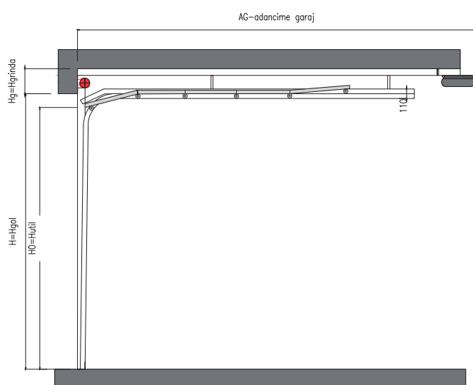
SECȚIUNE VERTICALĂ UȘA SECȚIONALĂ MODEL Lego
