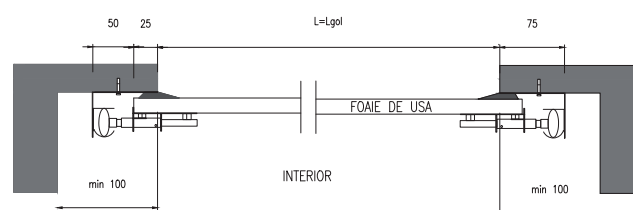
SECȚIUNE ORIZONTALĂ UȘA SECȚIONALĂ
