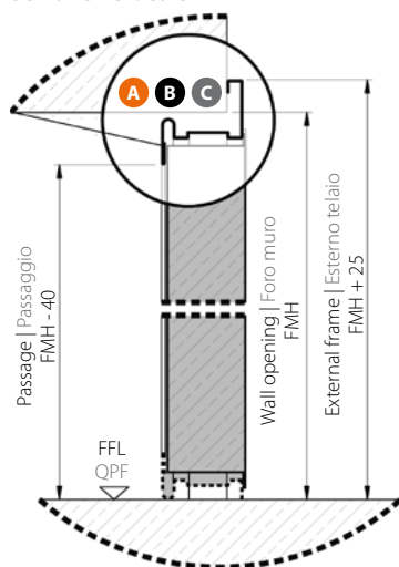
Vertical section Sezione verticale
