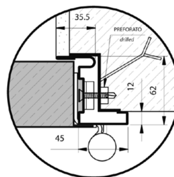
Sub-Frame Falso telaio
